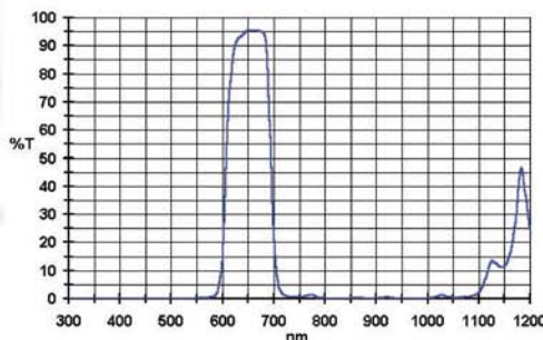
Spektrale Transmissionskurve UV/IR-Sperrfilter & BAADER RG 610 Rotfilter, kombiniert als H- \alpha Passfilter
