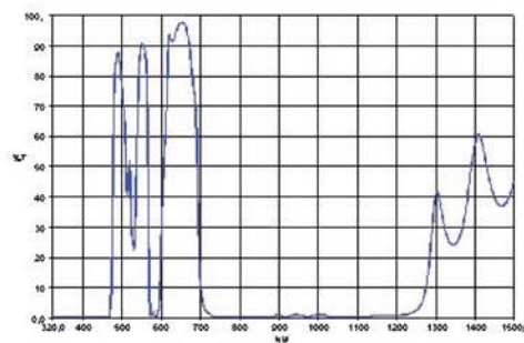
Spektrale Transmissionskurve UV/IR-Sperrfilter & BAADER Kontrast-Booster: wirkt wie ein RGB-Verstärker!
